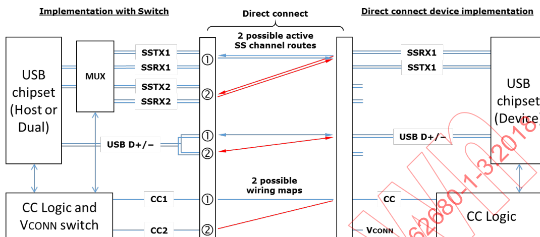
Figure 4-4 – Modèle logique pour les ports basés sur USB Type-C du dispositif à connexion directe
