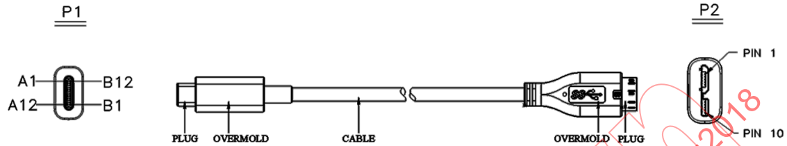
Figure 3-29 – Ensemble de câbles USB Type-C vers USB 3.1 Micro-B
