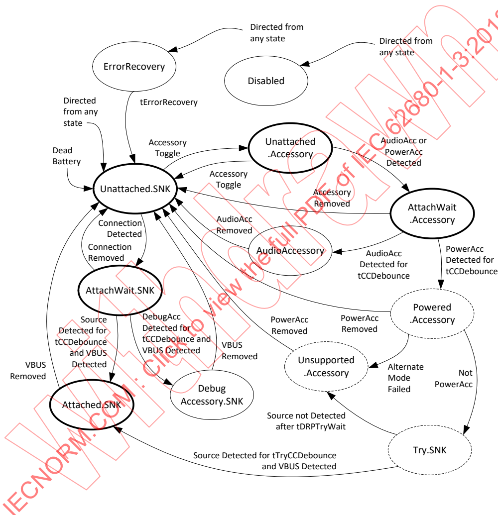
Figure 4-14 – Diagramme d'états de connexion: Collecteur avec prise en charge des modes accessoires
