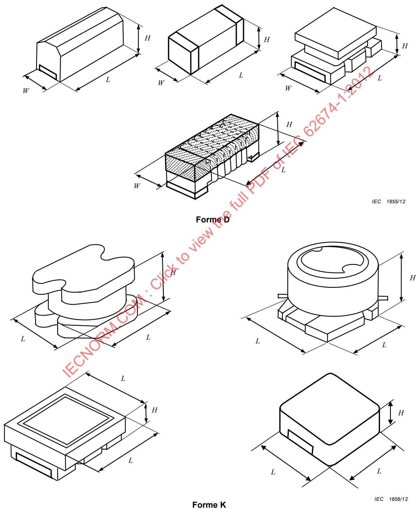
Figure 1 – Formes d'inductances et de perles de ferrite (exemples)
