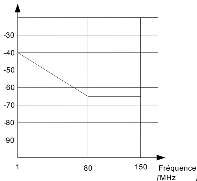
Figure 3 – Maximum des composantes haute fréquence de la tension de sortie
