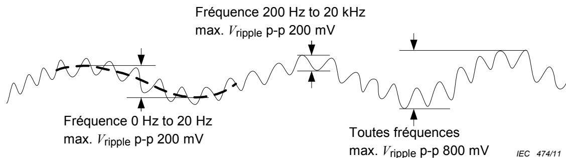
Figure 2 – Ondulation maximale crête à crête de la tension
