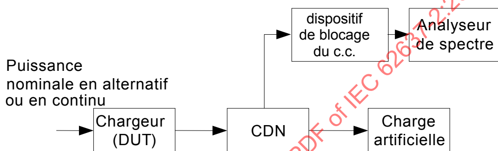
Figure 4 – Montage d'essai des composantes haute fréquence de la tension de sortie
