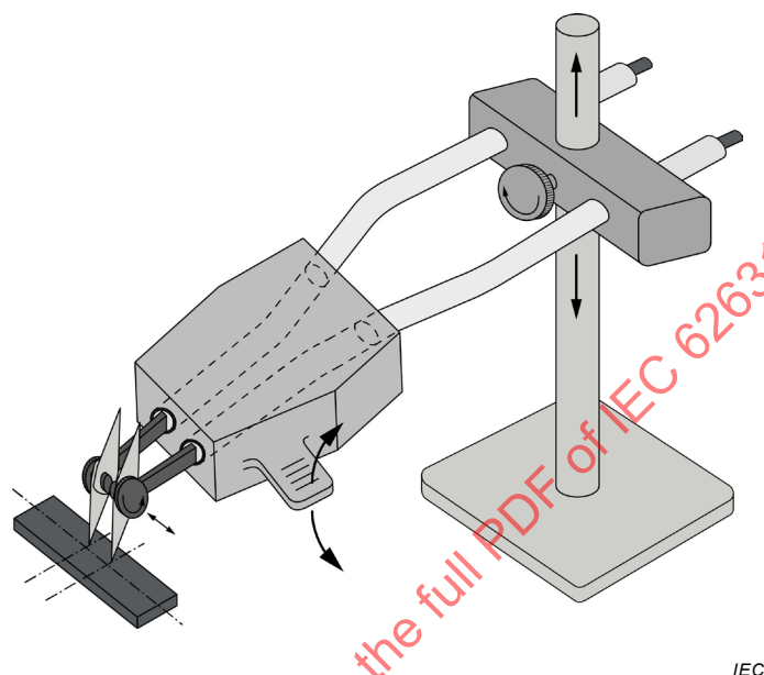
Figure 2 – Electrode collectrice pour l'arrangement d'électrodes B
