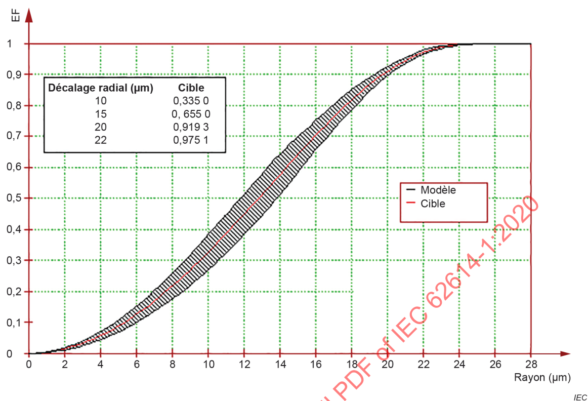
Figure 1 – Représentation du modèle EF pour un câblage avec fibre d'un diamètre de cœur de 50 μm à 850 nm
