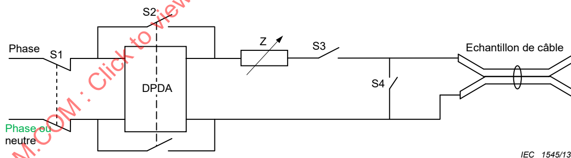
Figure 6 – Circuit d'essai pour essais de défaut d'arc en parallèle
