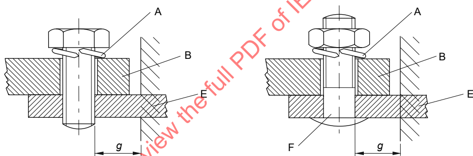
Figure IB.3 – Exemples de bornes à plaquette
