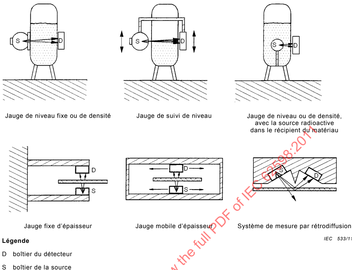
Figure 1 – Disposition schématique des jauges de Catégorie A
