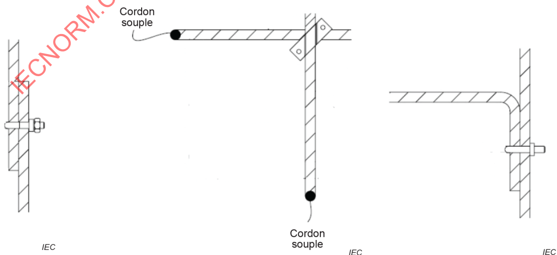
Figure 5 – Montage de base des échantillons avec connexion par serrage de tiges de renfort
