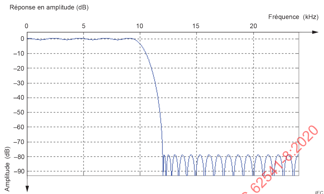
Figure 3 – Représentation graphique d'un YArrayItem
