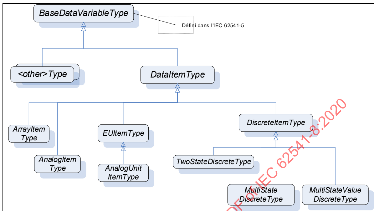
Figure 2 – Hiérarchie du VariableType DataItem
