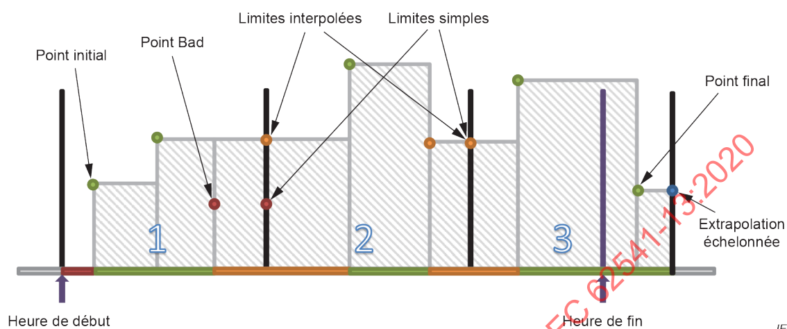
Figure 3 – Variable avec Stepped = True et Valeurs limites interpolées
