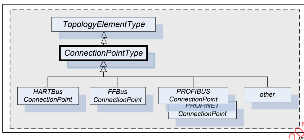
Figure 16 – Exemple de hiérarchie de ConnectionPointType
