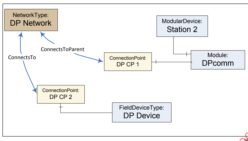
Figure 20 – Exemple avec les Références ConnectsTo et ConnectsToParent
