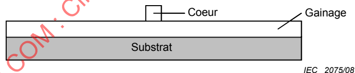
Figure 1c – Exemple de carte à guides d'ondes en canaux – Type à nervures
