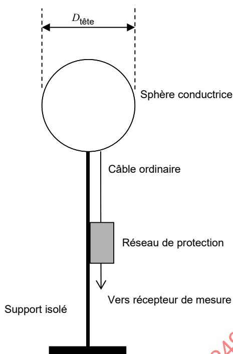
Figure 2 – Tête d'essai Van der Hoofden
