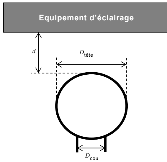
Figure D.6 – Distances entre la tête et le montage de mesure
