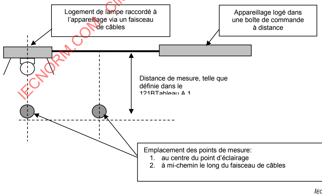
Figure B.8 – Emplacement des points de mesure d'un équipement d'éclairage muni d'un appareillage à distance
