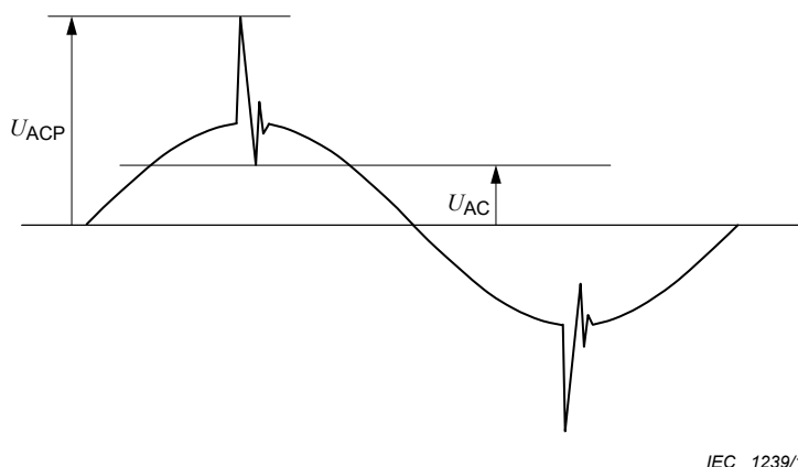
Figure A.20 – Forme d'onde type pour la tension de fonctionnement c.a.
