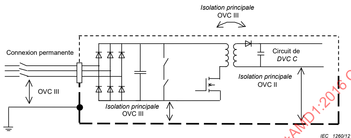
Figure I.12 – Evaluation de l' isolation principale pour les circuits connectés et non connectés directement au réseau
