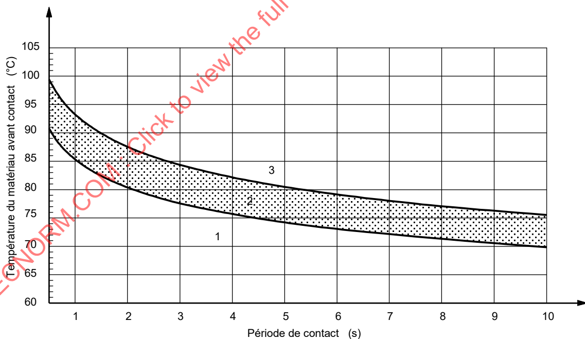
Figure J.4 – Répartition du seuil de brûlure lorsque la peau est en contact avec une surface lisse brûlante constituée de céramique, verre et pierres
