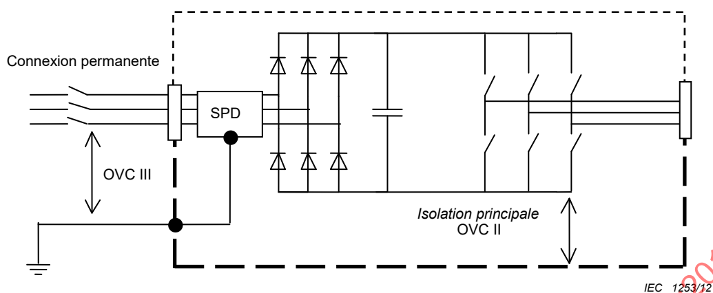
Figure I.5 – Évaluation de l' isolation principale pour les circuits connectés au réseau où des dispositifs de protection contre les surtensions (SPD) internes sont utilisés
