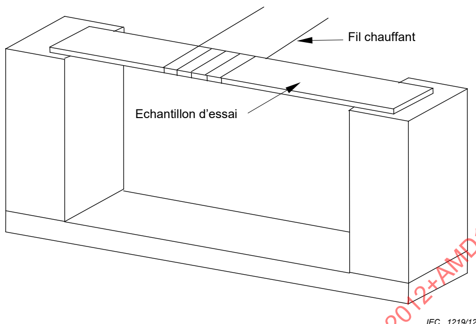
Figure 14 – Montage pour essai d'inflammation au fil chaud
