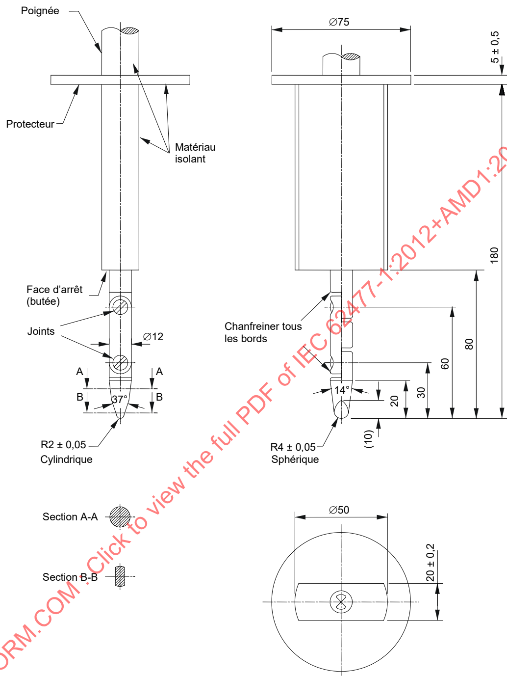
Figure M.2 – Doigt d'essai assemblé (IPXXB)
