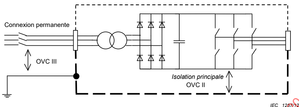
Figure I.9 – Evaluation de l' isolation principale pour les circuits non connectés directement au réseau
