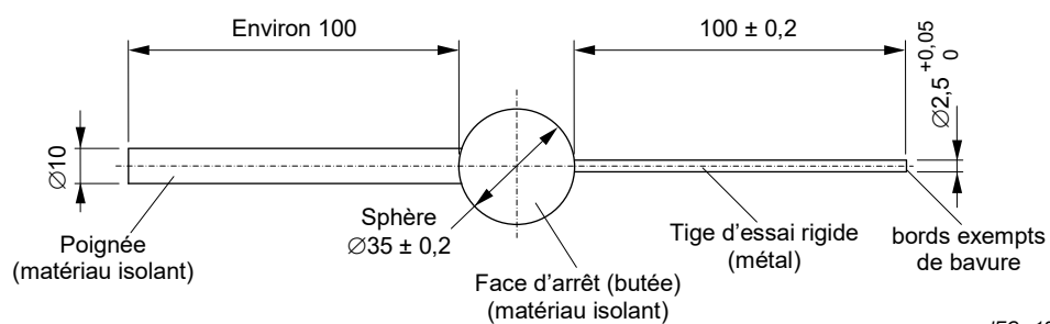
Figure M.3 – Tige d'essai de 2,5 mm (IP3X)
