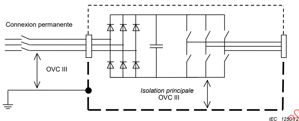
Figure I.2 – Evaluation de l' isolation principale pour les circuits connectés au réseau
