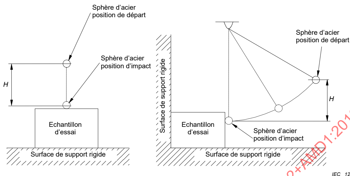
Figure 9 – Essai de choc utilisant la sphère d'acier
