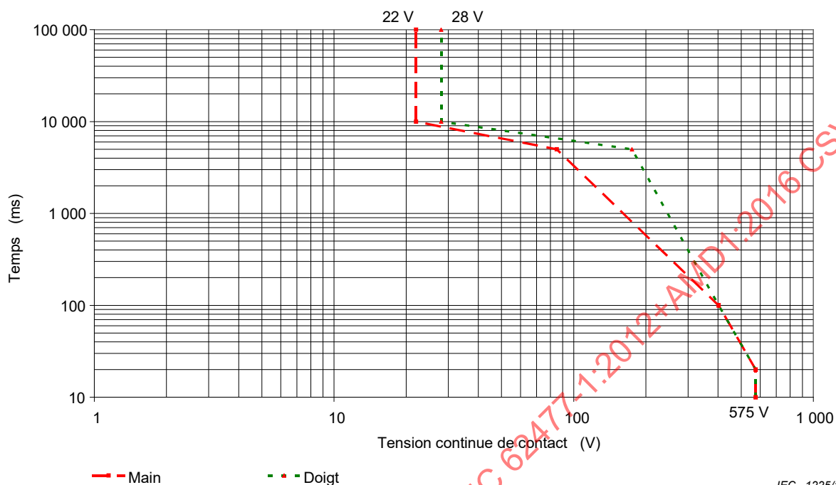
Figure A.5 – Zones temps-tension continue de contact pour la condition de peau humide
