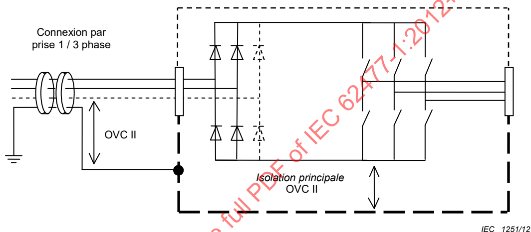
Figure I.3 – Evaluation de l' isolation principale pour les matériels mono et triphasés non connectés en permanence au réseau
