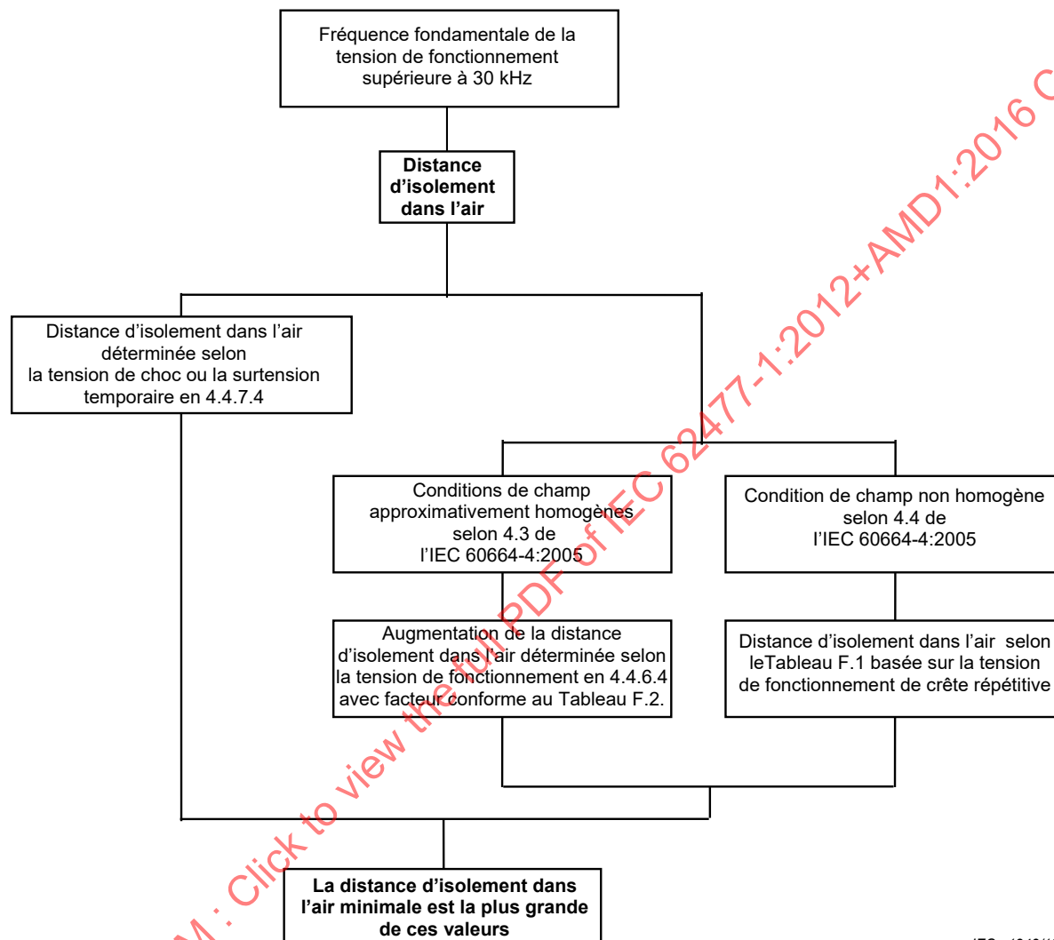
Figure F.1 – Schéma de dimensionnement des distances d'isolement dans l'air
