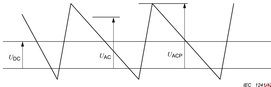
Figure A.22 – Forme d'onde type pour la tension de fonctionnement pulsante
