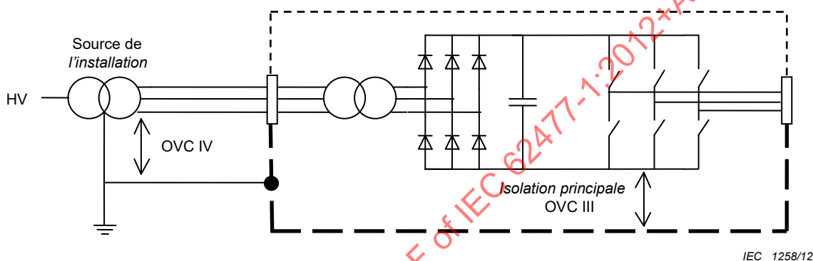
Figure I.10 – Evaluation de l' isolation principale pour les circuits non connectés directement au réseau
