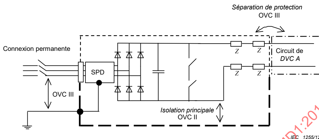
Figure I.7 – Exemple d'évaluation de la séparation de protection pour les circuits connectés au réseau où des dispositifs de protection contre les surtensions (SPD) internes sont utilisés
