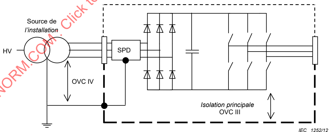
Figure I.4 – Évaluation de l' isolation principale pour les circuits connectés à la source du réseau de l'installation où des dispositifs de protection contre les surtensions (SPD) internes sont utilisés
