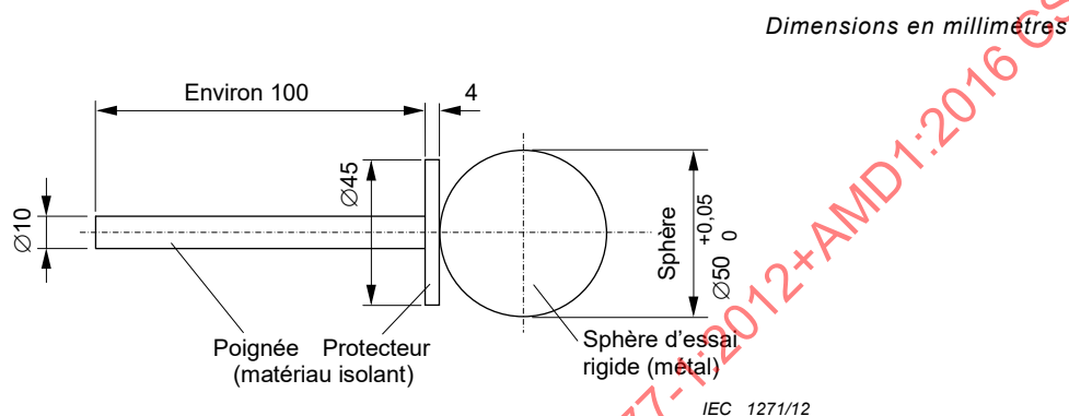
Figure M.1 – Sphère d'essai de 50 mm (IPXXA)
