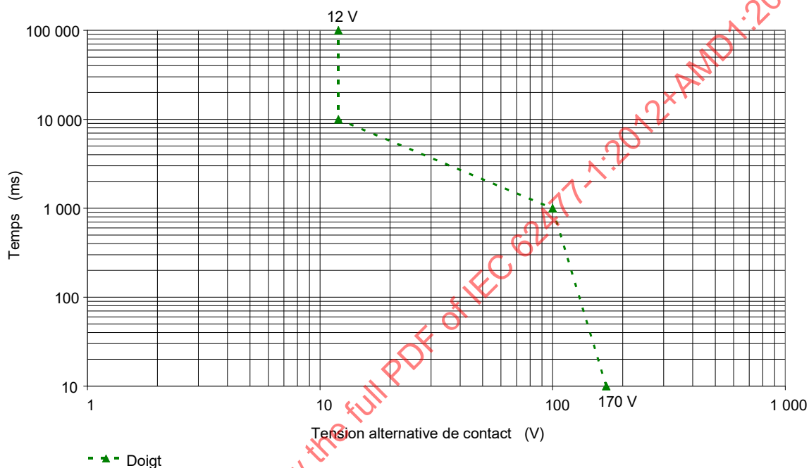
Figure A.18 – Zones temps-tension alternative de contact pour la condition de peau sèche
