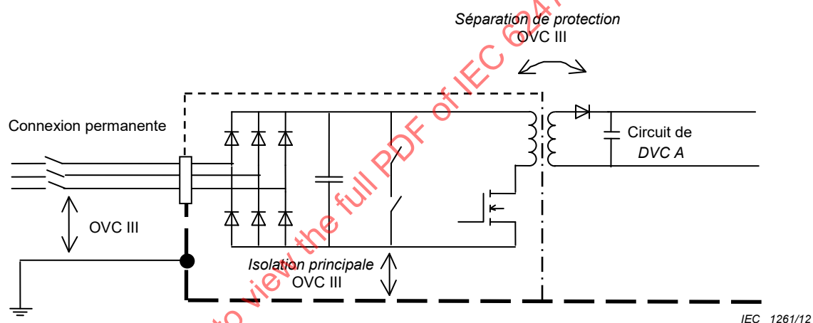
Figure I.13 – Evaluation de l' isolation pour un circuit accessible de CTD A
