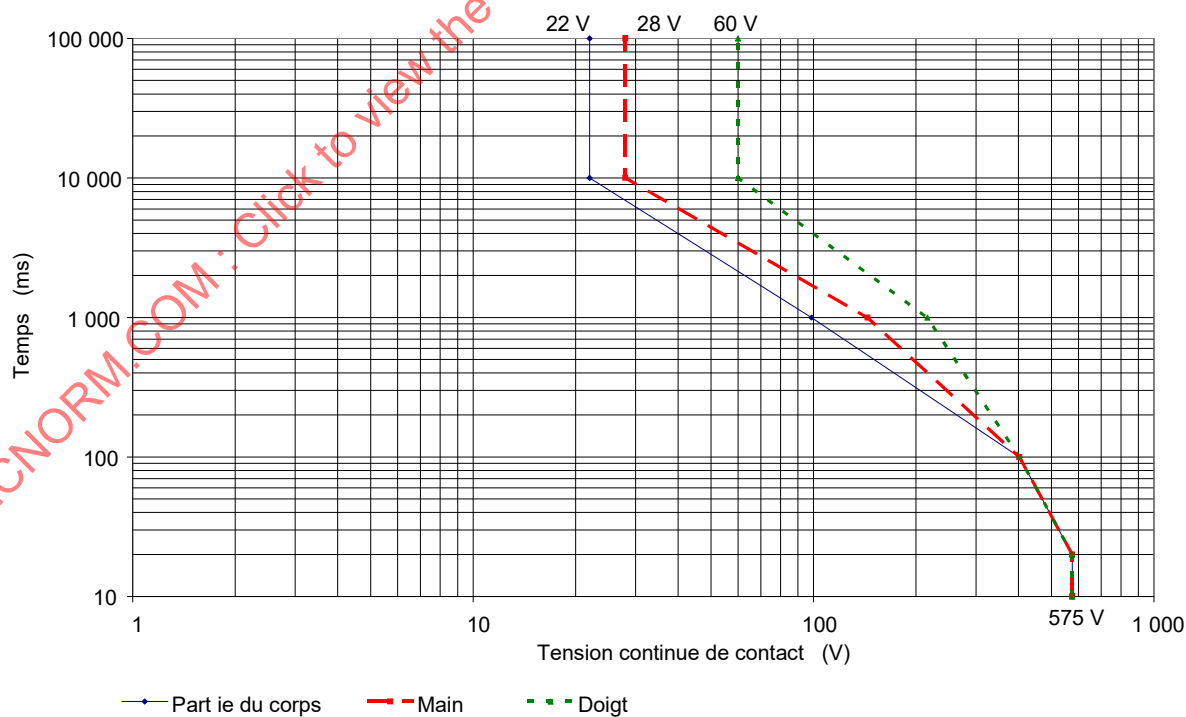
Figure A.4 – Zones temps-tension continue de contact pour la condition de peau sèche
