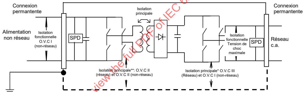
Figure I.14 – CEP avec réseau et non-réseau sans séparation galvanique
