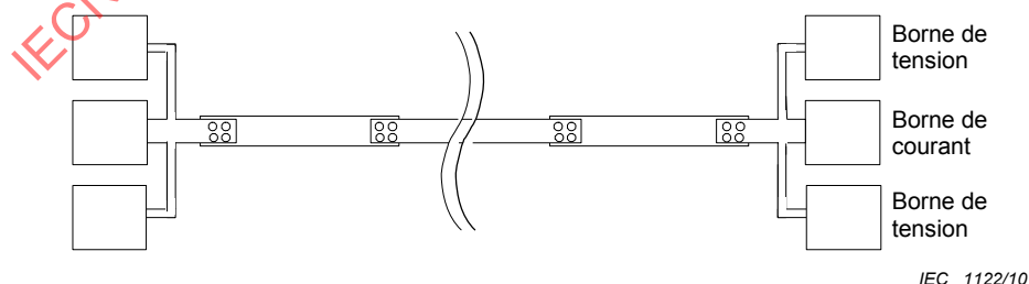
Figure 2 – TEG d'évaluation de l'électromigration pour trou de liaison
