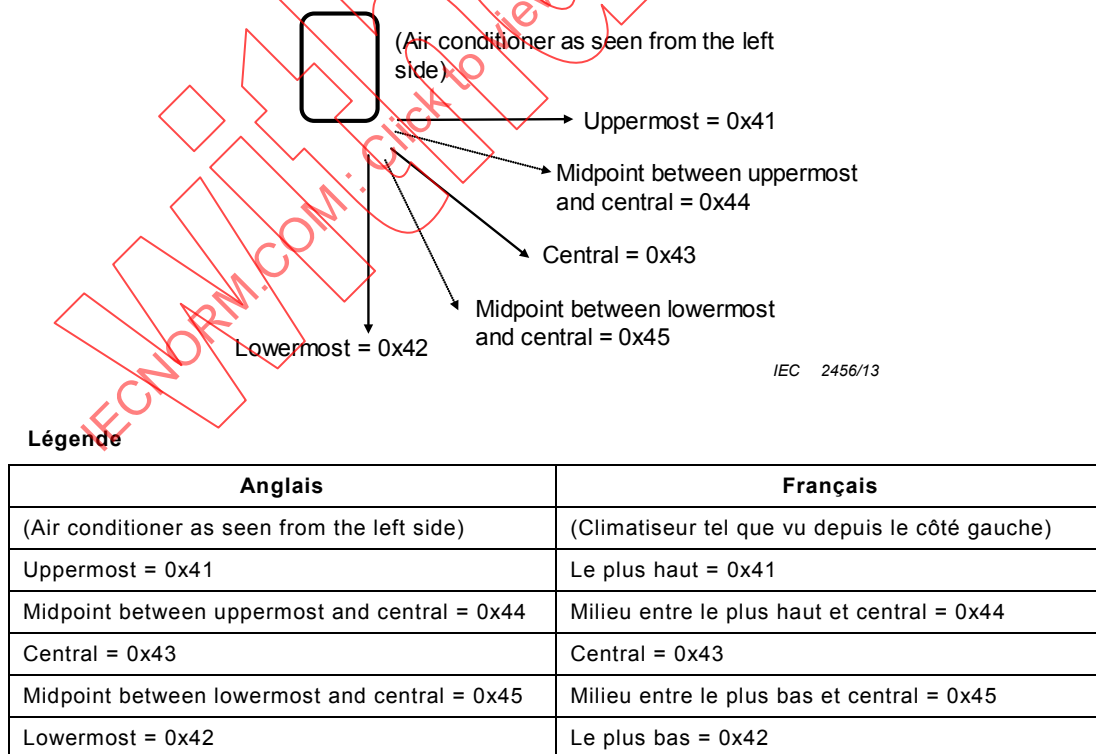
Figure 49 – Réglage de la direction de débit d'air (vertical)
