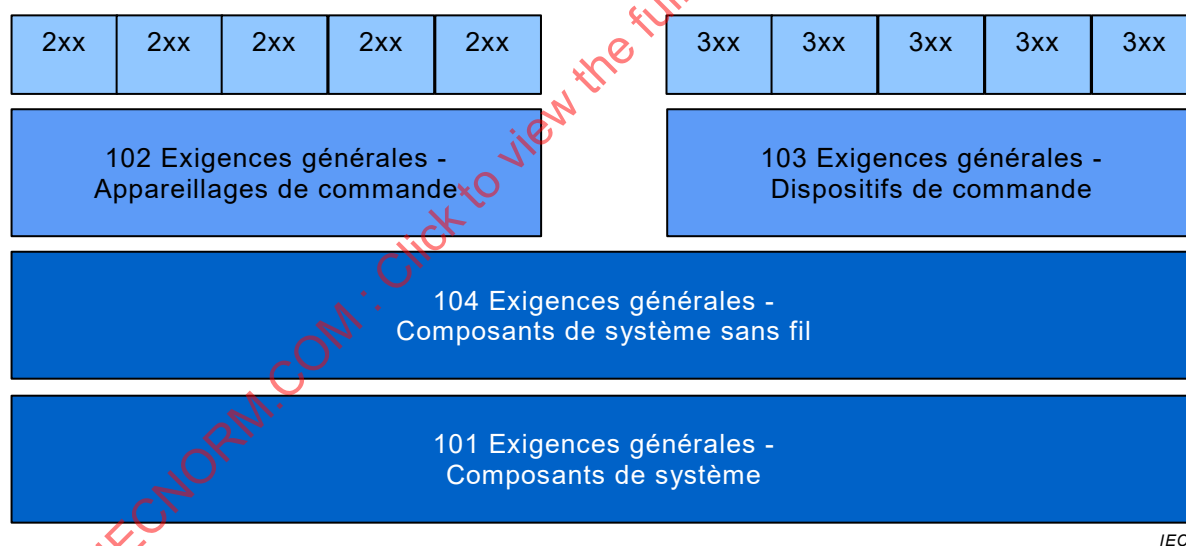
Figure 1 – Présentation graphique générale de l'IEC 62386
