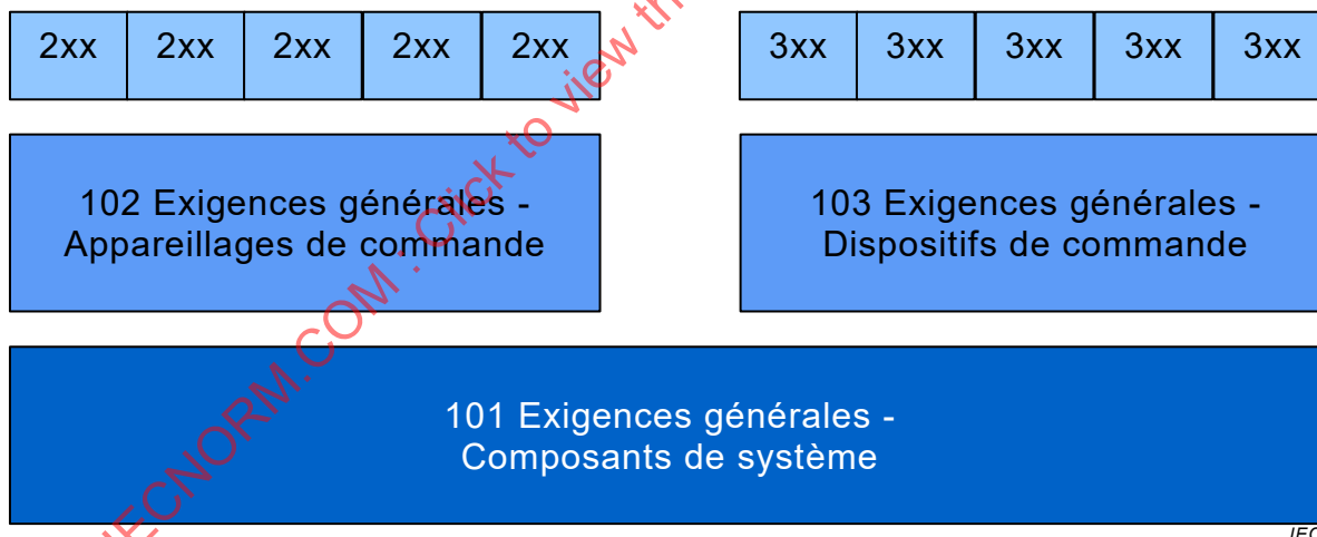
Figure 1 – Vue d'ensemble graphique de l'IEC 62386
