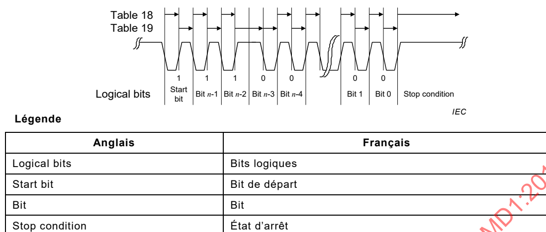
Figure 14 – Exemple de décision de cadencement du récepteur
