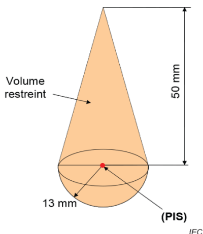
Figure 37 – Exigences minimales de séparation d'une source potentielle d'incendie (PIS)
