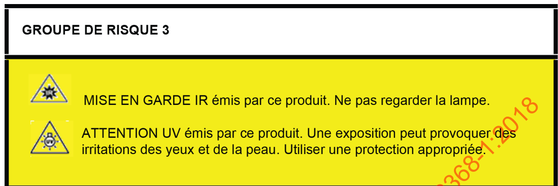
Figure 50 – Exemple d'étiquette de mise en garde pour une lampe avec plusieurs zones dangereuses du spectre
