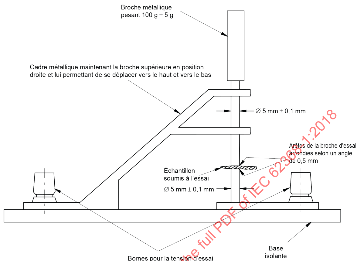
Figure 29 – Exemple d'instrument d'essai de rigidité diélectrique pour une isolation solide
