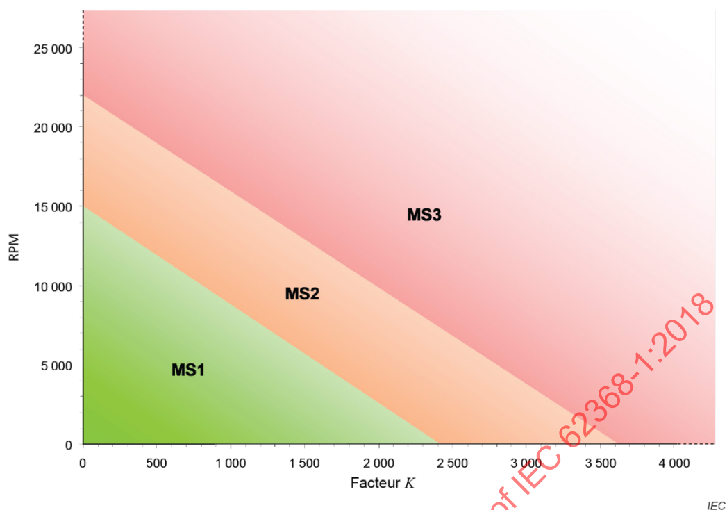
Figure 45 – Limites pour les pales mobiles de ventilateurs en matériaux autres que le plastique
