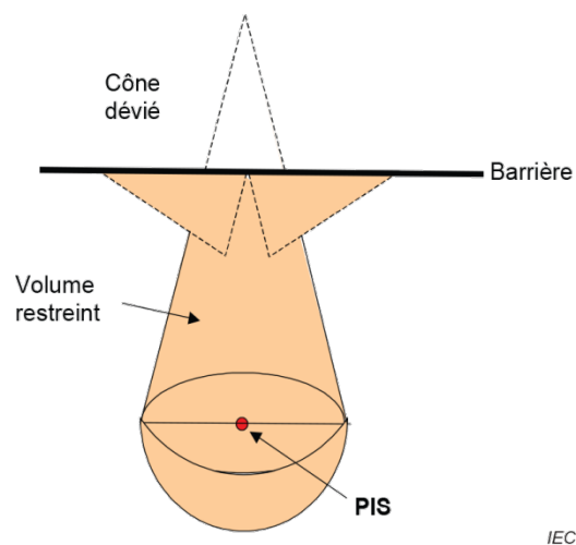
Figure 39b – Représentation d'une barrière horizontale
