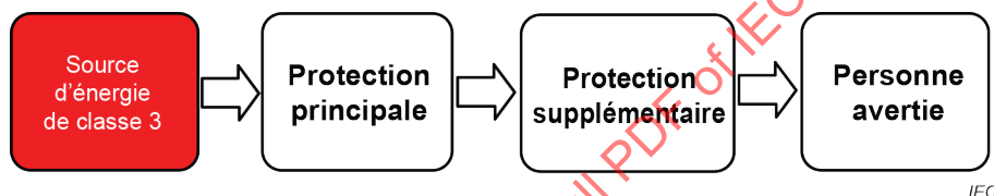
Figure 15 – Modèle pour protéger une personne avertie contre une source d'énergie de classe 3
