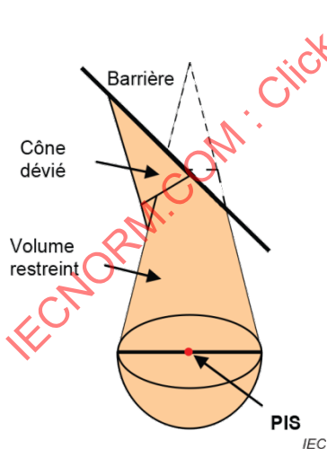
Figure 39a – Représentation d'une barrière oblique
