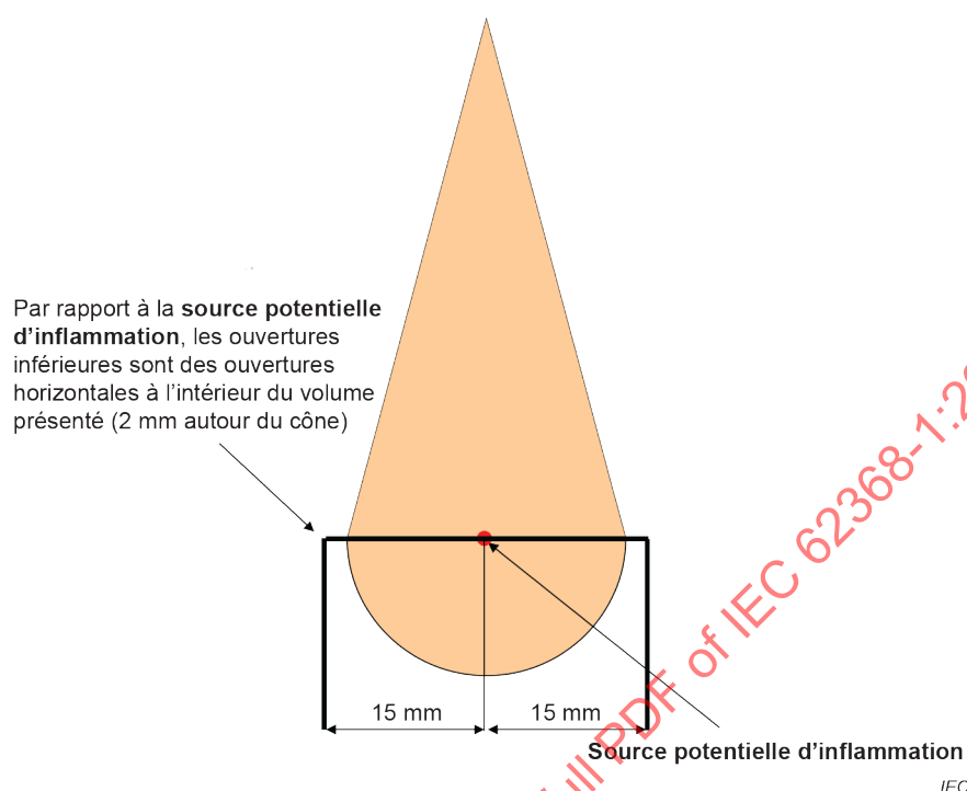
Figure 42 – Ouvertures dans le fond
