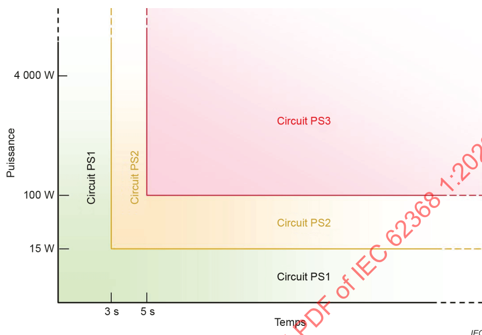
Figure 36 – Représentation de la classification des sources de puissance
