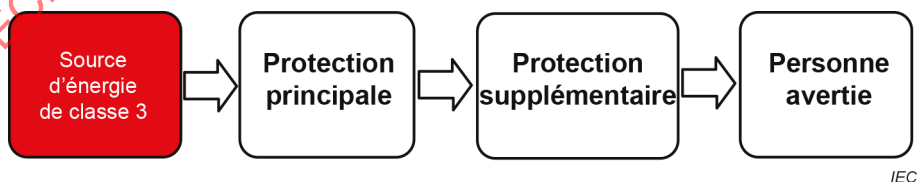
Figure 15 – Modèle de protection d'une personne avertie contre une source d'énergie de classe 3
