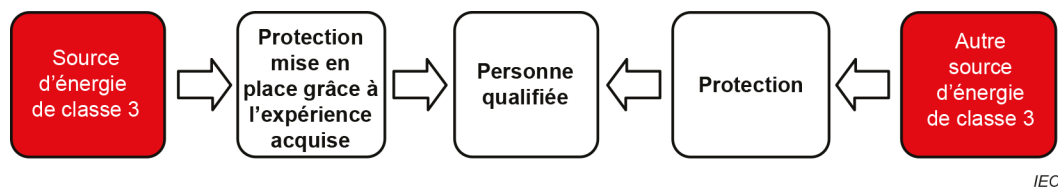
Figure 19 – Modèle de protection d'une personne qualifiée contre des sources d'énergie de classe 3 dans les conditions d'entretien de l'équipement
