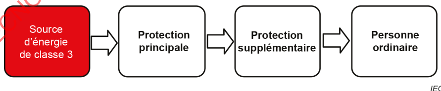
Figure 12 – Modèle de protection d'une personne ordinaire contre une source d'énergie de classe 3
