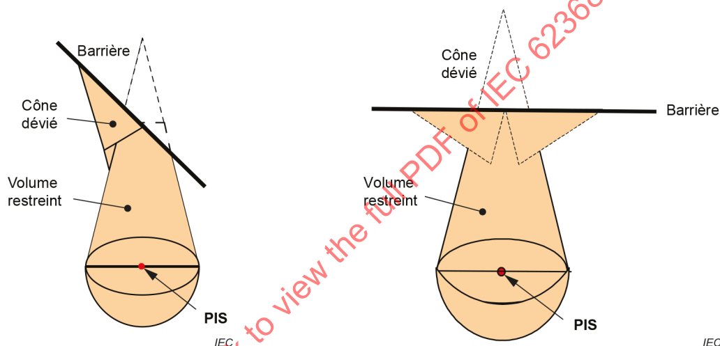
Figure 39a – Représentation d'une barrière oblique
