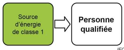
Figure 16 – Modèle de protection d'une personne qualifiée contre une source d'énergie de classe 1
