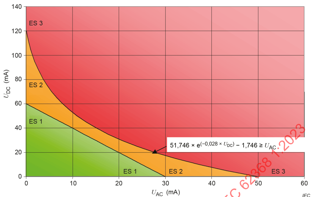
Figure 23 – Valeurs maximales pour les tensions mixtes en courant alternatif et en courant continu
