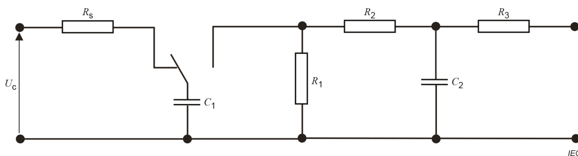
Figure D.1 – Générateur de tension de choc de 1,2/50 \mu\text{s} et 10/700 \mu\text{s}
