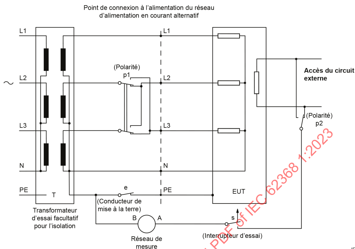
Figure 33 – Circuit d'essai pour le courant de contact des équipements triphasés
