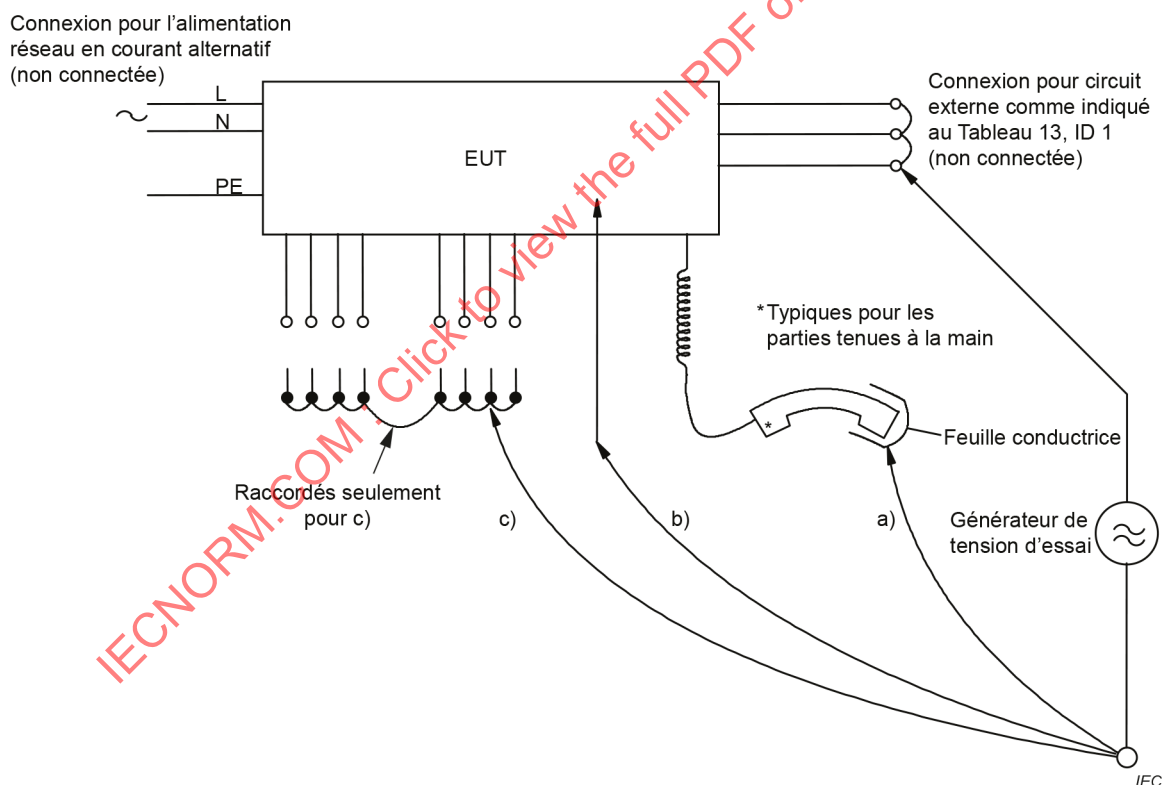
Figure 30 – Points d'application de la tension d'essai
