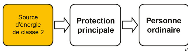
Figure 10 – Modèle de protection d'une personne ordinaire contre une source d'énergie de classe 2
