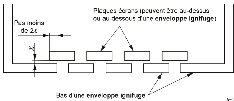
Figure 43 – Construction avec plaque-écran
