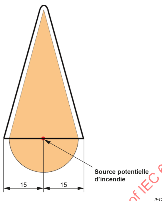
Figure 41 – Ouvertures sur le dessus
