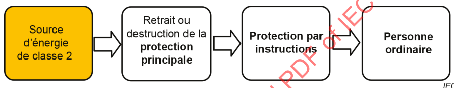
Figure 11 – Modèle de protection d'une personne ordinaire contre une source d'énergie de classe 2 dans les conditions d'entretien par une personne ordinaire
