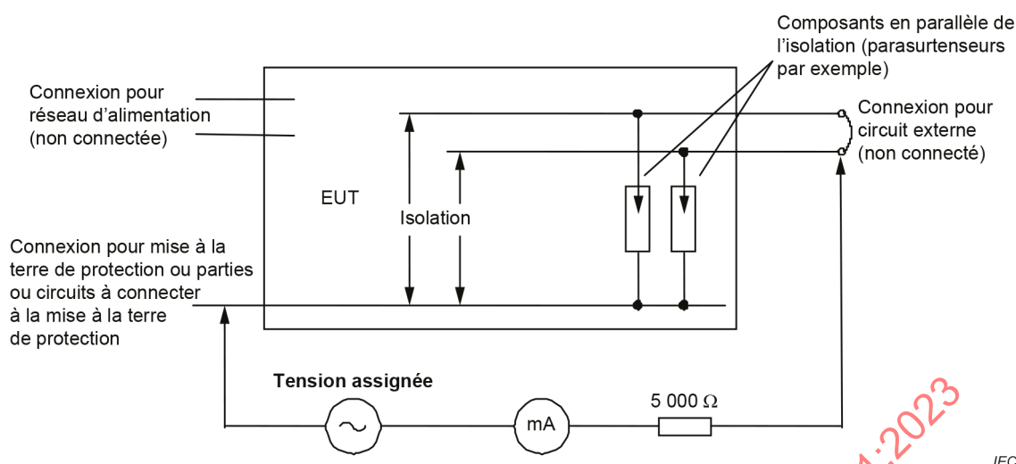
Figure 31 – Essai de séparation entre un circuit externe et la terre
