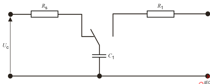
Figure D.2 – Circuit du générateur d'essai pour l'interface d'antenne
