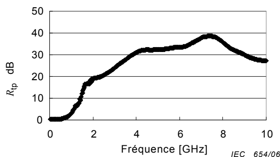
Figure 11c – R_{tp} calculé à partir de S_{11M} et S_{21M}
