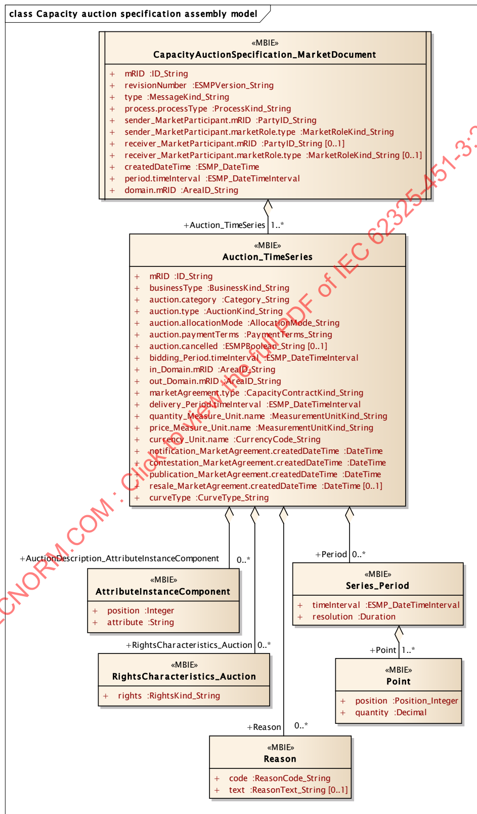
Figure 12 – Modèle d'assemblage de spécification de vente aux enchères de capacité
