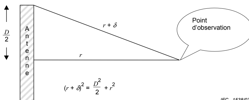
Figure A.1 – Géométrie de l'antenne dont la plus grande dimension linéaire est D
