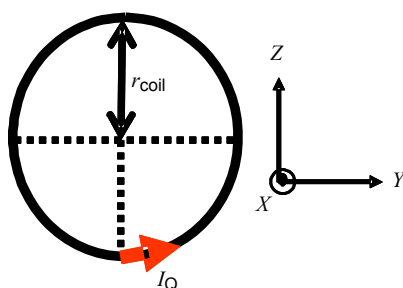
Figure C.5 – Schéma de bobine circulaire
