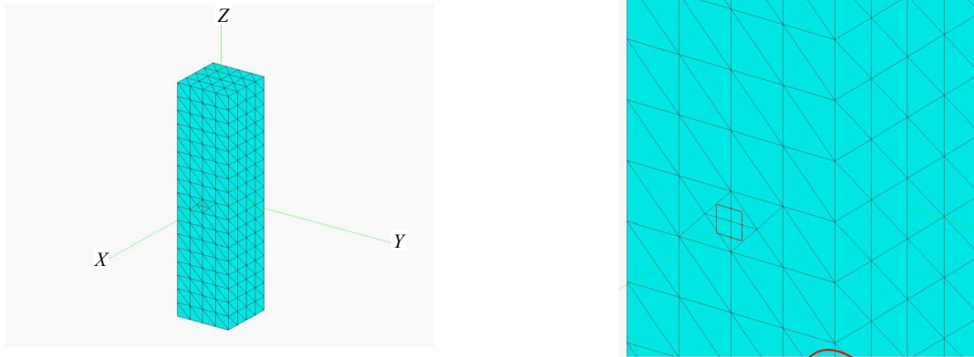
Figure C.7 – Situation d'essai pour validation – Boucle de courant en face d'un cube
