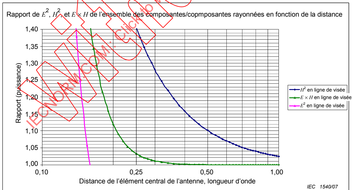
Figure A.3 – Rapport des composantes de champ de E^2 , H^2 , et E \times H
