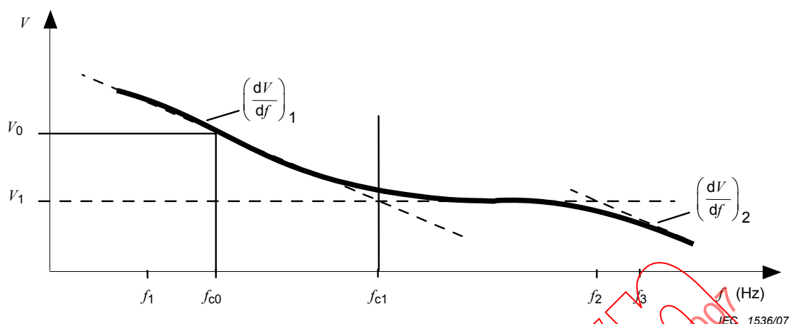
Figure 3 – Dépendance par rapport à la fréquence des niveaux de référence V avec lissage des arêtes
