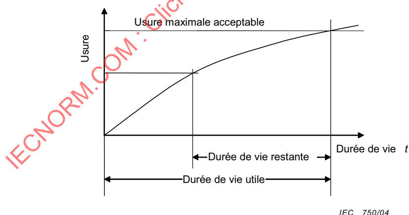
Figure A.1 – Exemple pour la détermination de la durée de vie restante des composants
