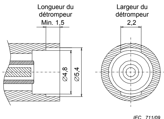
Figure 8 – Détrompeur mécanique (large et type de détrompeur 2)
