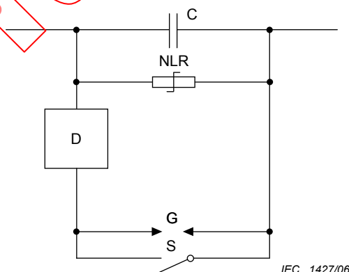
Éclateur double
