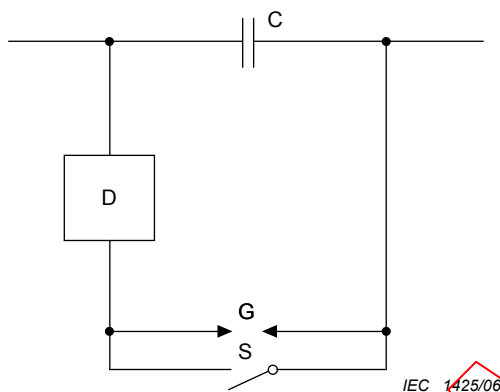
Éclateur simple
