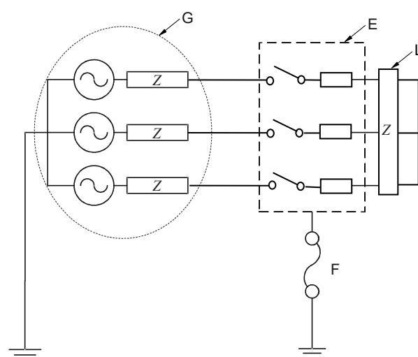
Figure 2a – Circuit d'essai avec charge
