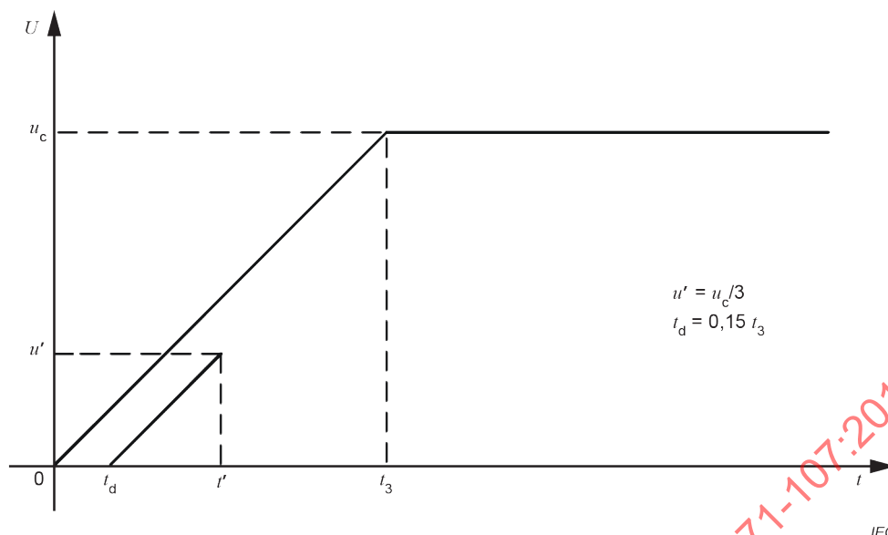
Figure 3 – Représentation d'une TTR spécifiée par un tracé de référence à deux paramètres et un retard
