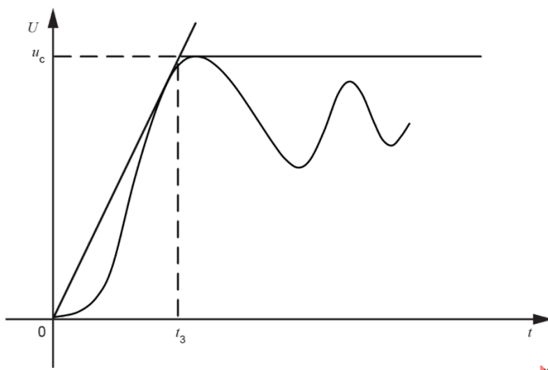
Figure 4 – Exemple d'enveloppe à deux paramètres pour une TTR
