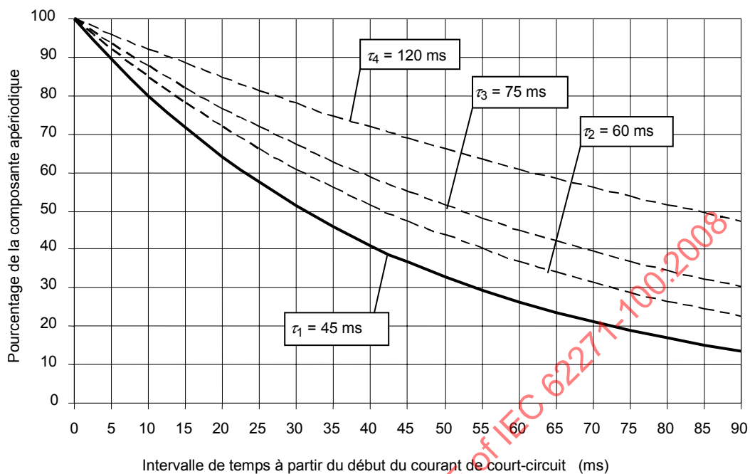
Figure 9 – Pourcentage de la composante apériodique en fonction de l'intervalle de temps à partir du début du courant de court-circuit pour la constante de temps normale \tau_1 et pour les constantes de temps \tau_2 , \tau_3 et \tau_4 des applications particulières
