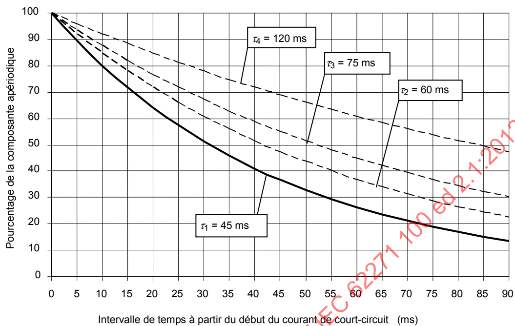
Figure 9 – Pourcentage de la composante aperiodique en fonction de l'intervalle de temps à partir du début du courant de court-circuit pour les différentes constantes de temps normale \tau_1 et pour les constantes de temps \tau_2 , \tau_3 et \tau_4 des applications particulières
