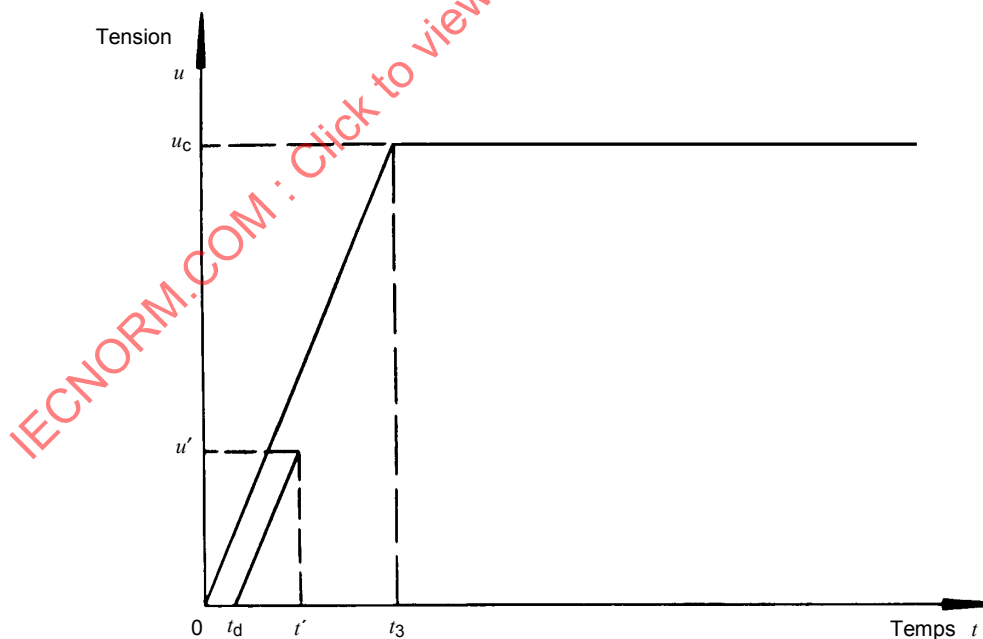
Figure 11 – Représentation d'une TTR spécifiée par un tracé de référence à deux paramètres et par un segment de droite définissant un retard
