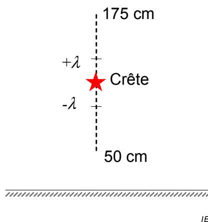
Figure I.2 – Moyennage spatial relatif à une hauteur de champ d'intensité maximale
