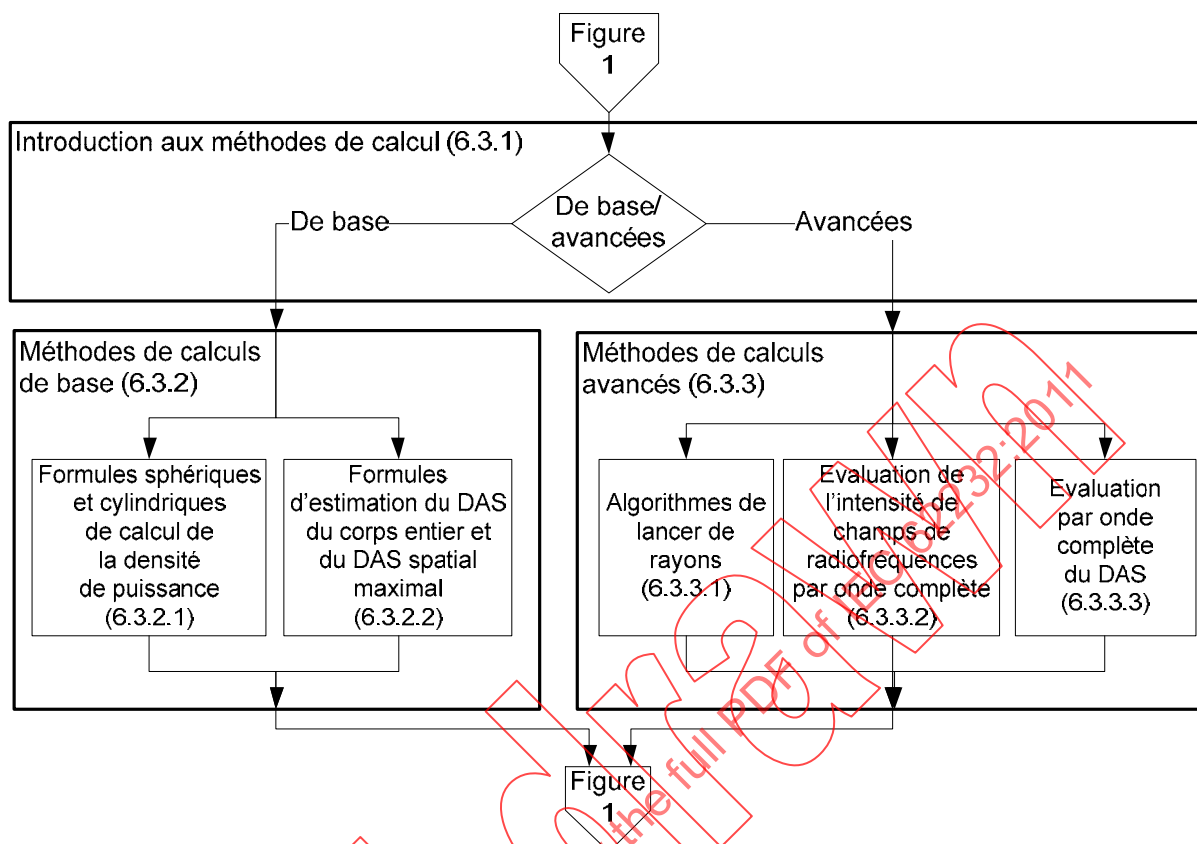
Figure 4 – Aperçu général des méthodes de calcul
