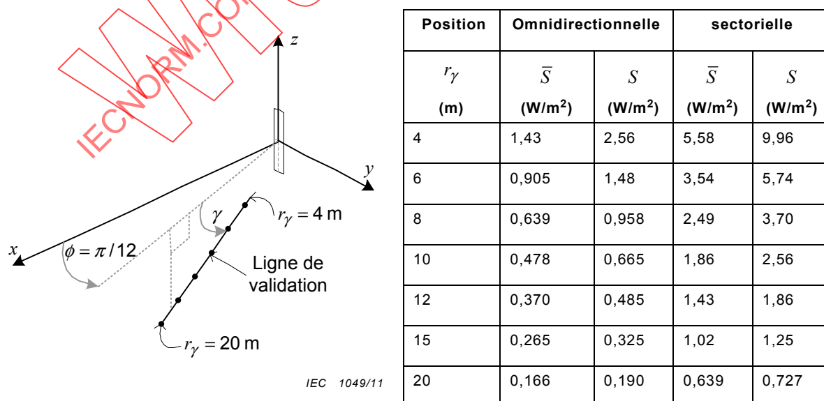
Figure H.1 – Résultats de référence pour des formules cylindriques
