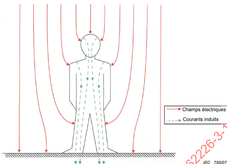
Figure 1 – Illustration du phénomène de courants induits par un champ électrique dans un corps humain debout sur le sol
