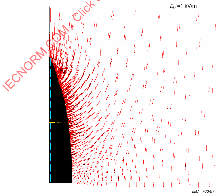
Figure 11 – Distorsion des lignes de champ électrique de fréquence industrielle à proximité du demi-sphéroïde conducteur
