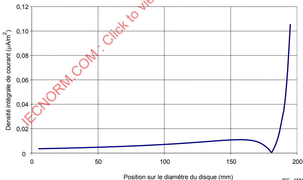
Figure D.7 – J_i = f[r] : Distribution de la densité intégrée de courant induit calculée le long du diamètre AA du disque (source: spire de rayon r = 10 mm, disque conducteur R = 100 mm, d = 5 mm)
