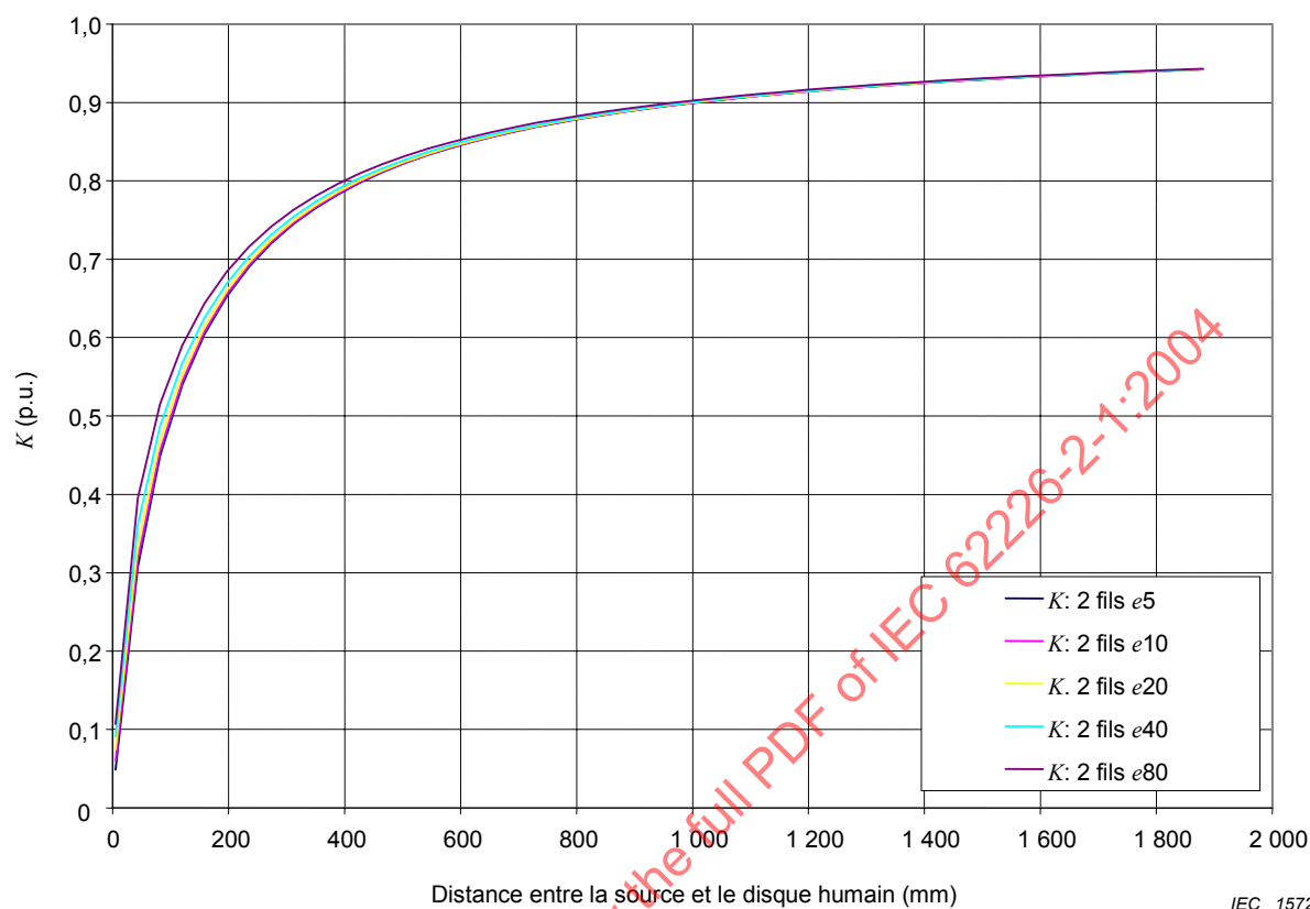
Figure C.7 – Courbes paramétriques du facteur K pour des distances jusqu'à 1 900 mm d'une source constituée de 2 fils parallèles parcourus par des courants équilibrés et pour différentes distances entre les 2 fils (disque homogène R = 100 mm)
