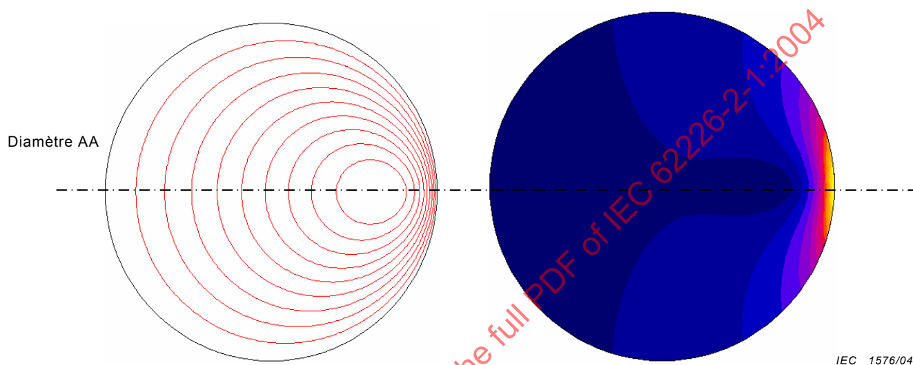
Figure D.2 – Lignes de densité de courant J et distribution de J dans le disque (source: spire de rayon r = 50 mm, disque conducteur R = 100 mm, d = 5 mm)
