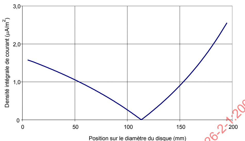
Figure B.6 – Distribution de la densité intégrée de courant induit le long du diamètre AA du disque (source: 1 fil, situé à d = 100 mm du bord du disque)
