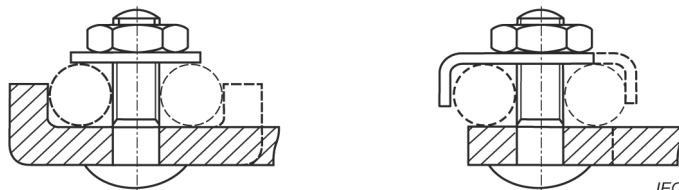
Figure 7 – Bornes à goujon fileté
