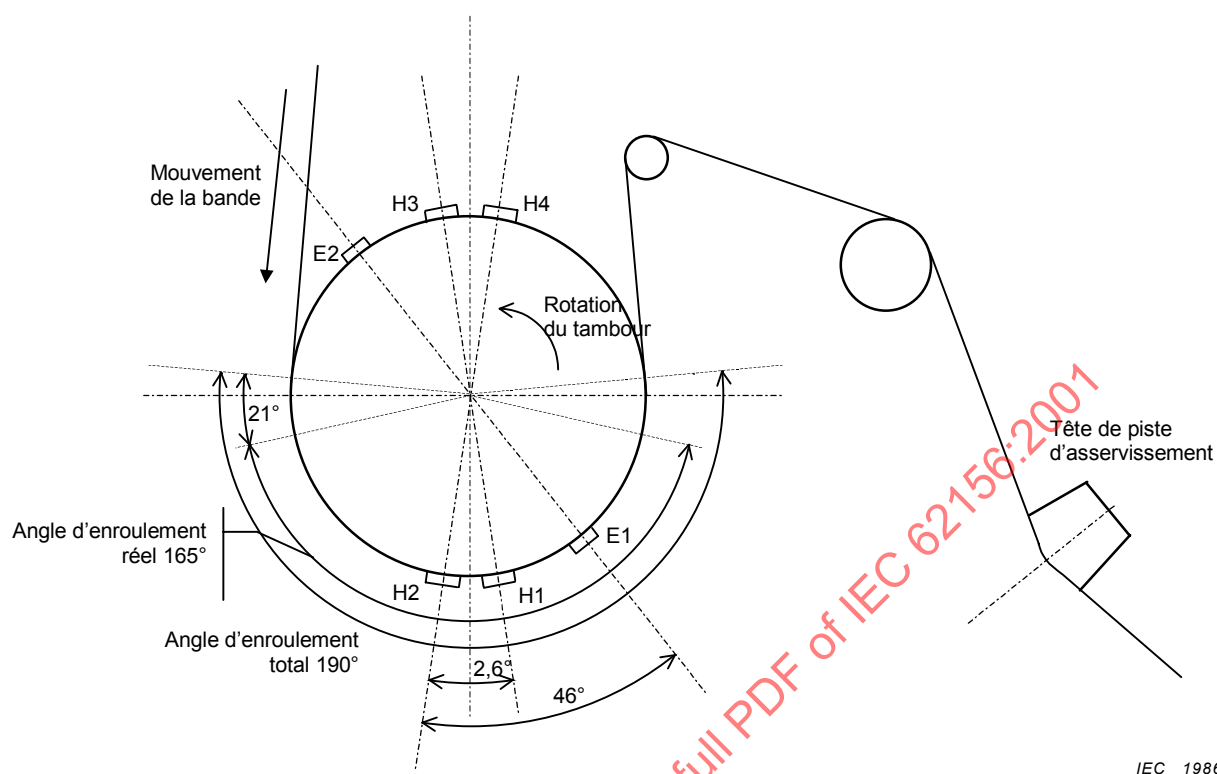
Figure 21a – Configuration possible du système de balayage (systèmes 525/60 et 625/50) – Vue de dessus
