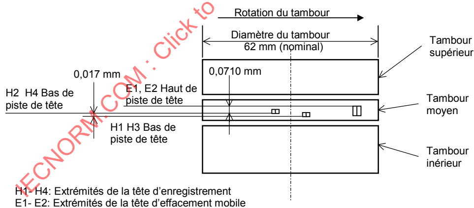
Figure 21b – Configuration possible du système de balayage (systèmes 525/60 et 625/50) – Vue latérale
