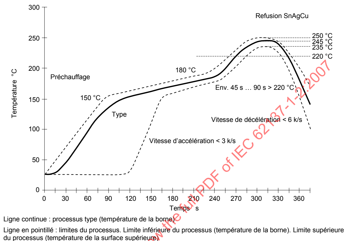
Figure 2 – Courbe type de brasage par refusion
