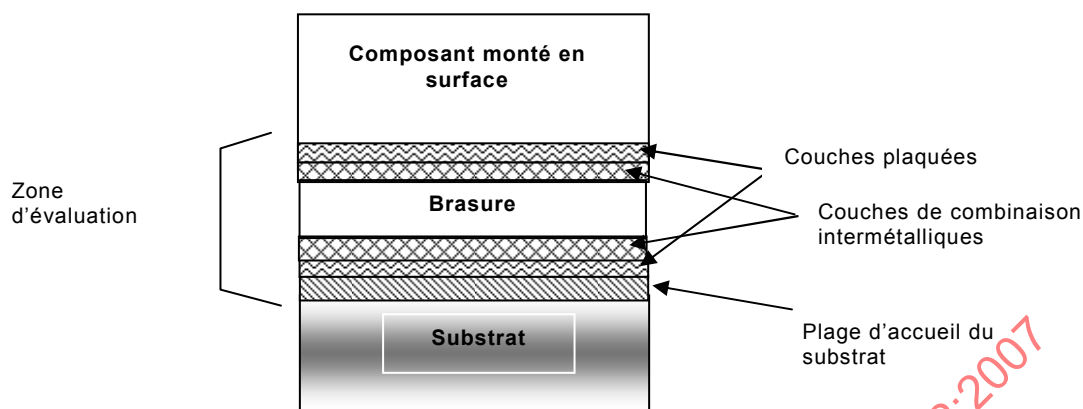
Figure 1 – Zone à évaluer lors de l'essai de résistance au cisaillement
