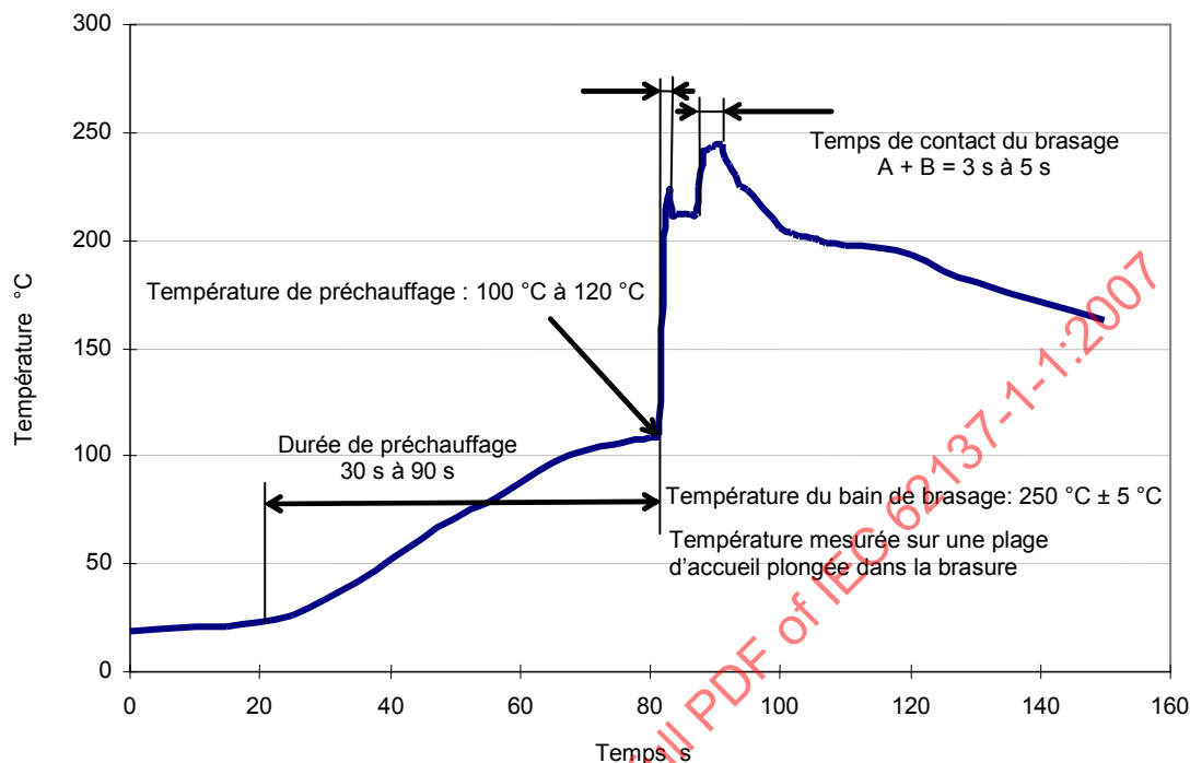
Figure 3 – Exemple de courbe de brasage à la vague (mesure réelle de la brasure à double vague)
