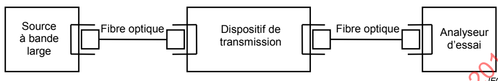
Figure 2 – Montage utilisant une source à large bande avec un dispositif de transmission
