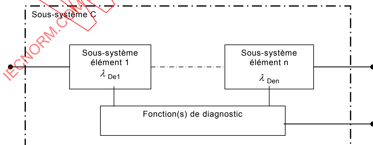
Figure 8 – Représentation logique d'un sous-système de type C
