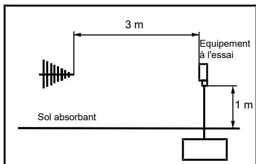
Figure D.1 – Montage d'essai pour l'essai d'immunité aux champs à fréquence radioélectrique électromagnétique HF
