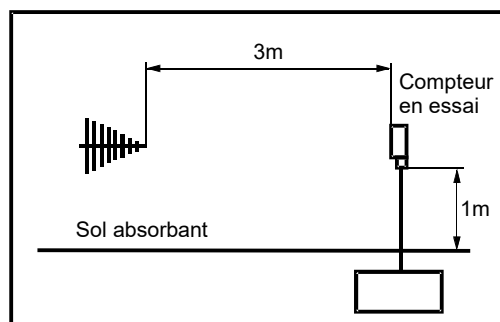
Figure E.1 – Montage d'essai pour l'essai de tenue aux champs électromagnétiques RF
