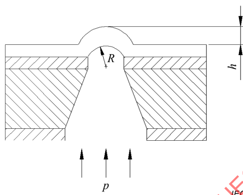
Figure 2 – Fenêtre à membrane bombée par la pression
