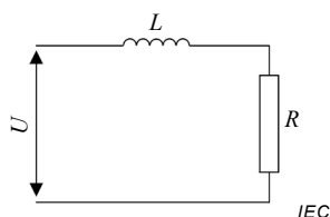
Figure BB.2 – Charge inductive-résistive de référence (série)
