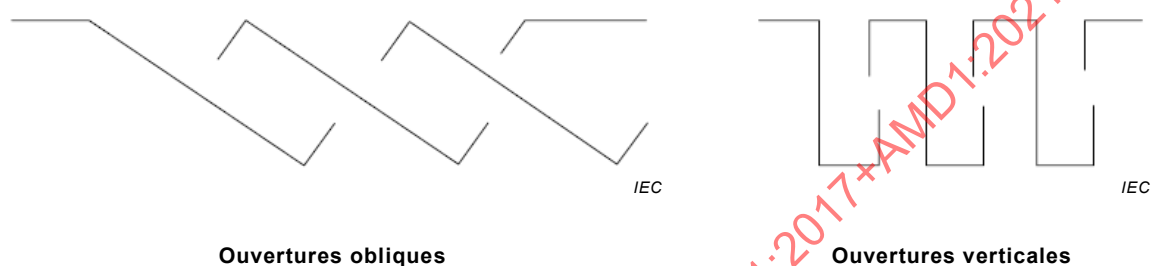
Figure 101 – Exemples de conceptions d'ouvertures destinées à empêcher l'accès vertical
