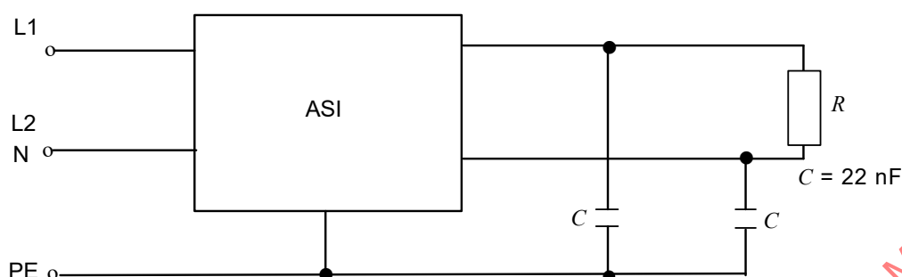
Figure 102 – Circuit d'essai pour variation du potentiel de référence induite par la charge – Sortie monophasée
