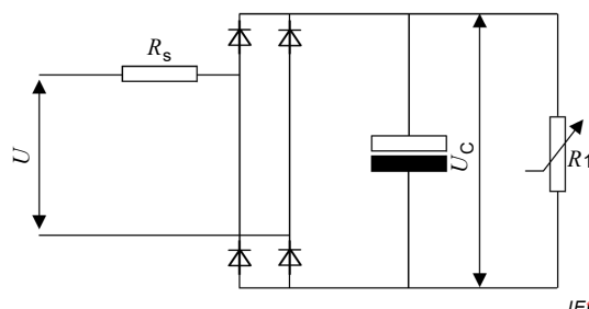
Figure BB.6 – Charge non linéaire de référence
