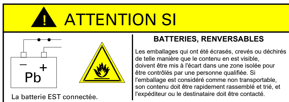
Figure DD.2 – Etiquette de sécurité pour les produits transportés avec leur batterie connectée
