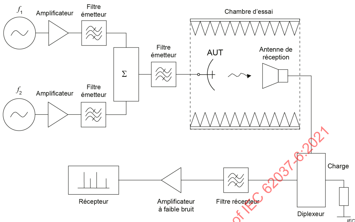
Figure 2 – Montage d'essai d'intermodulation passive directe de l'antenne
