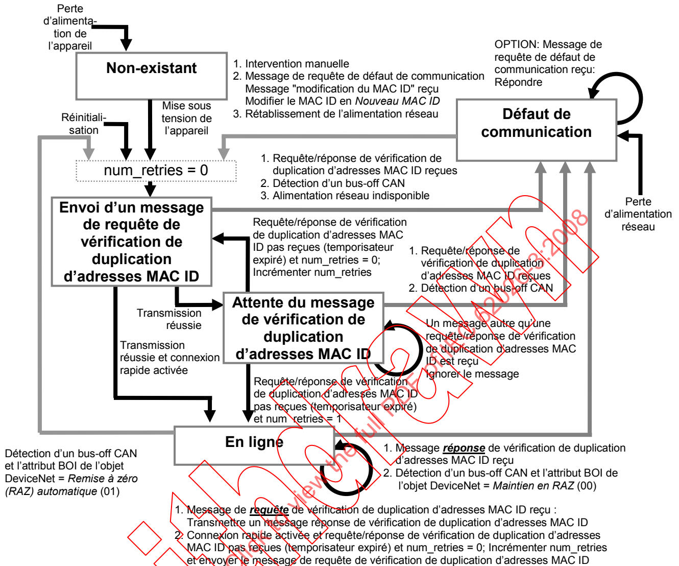
Figure 37 – Diagramme de la machine d'état d'accès à la liaison
