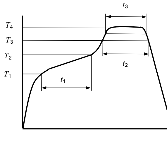
Figure 8 – Profil de température de refusion
