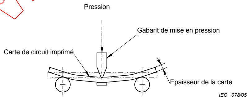
Figure 6 – Mise en pression
