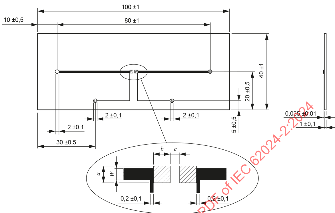
a) Exemple de carte à circuit imprimé pour les composants montés en surface (CMS) ( I classe A )
