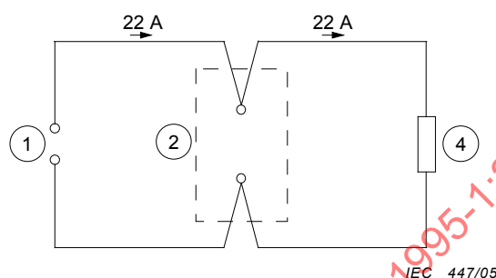
Figure 3b – Circuit pour essai 2
